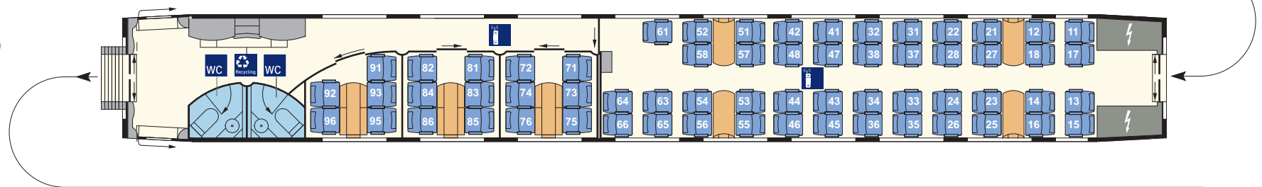
2. Kl.-Wagen (Bvmz 406.2) Nr. 27/37
