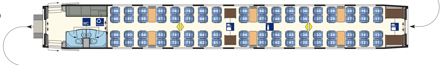
2. Kl.-Wagen (Bpmz 407.6) Nr. 22/32
