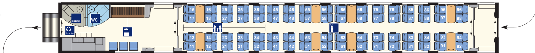
2. Kl.-Wagen (Bpmz 411.8) Nr. 24/34
